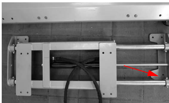
Fig. 12 Alignement de la pièce de décalage latéral
