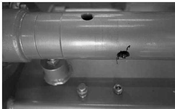
Fig. 30 Arbre de transmission avec orifice de contrôle et orifice de remplissage
