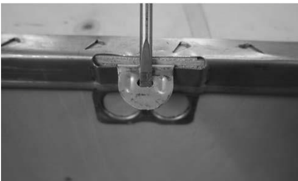
Fig. 3 Ouverture des fixations
