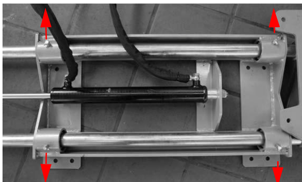
Fig. 11 Face inférieure avec alignement correct des graisseurs
