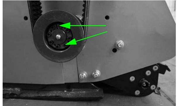
Fig. 28 Fixation de la poulie inférieure
