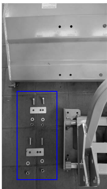
Fig. 14 Matériel de fixation pour pièce hydraulique de décalage latéral, côté gauche
